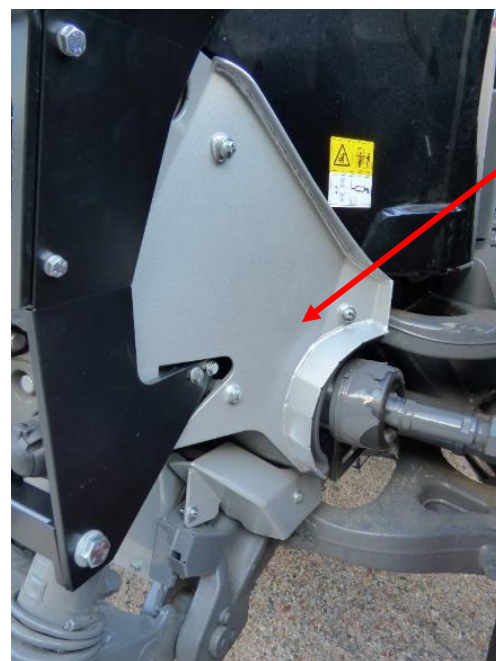
6 Protection vérin de direction avant
